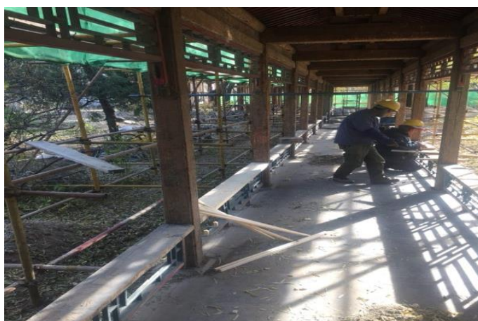
图 17 校景亭长廊等古建维修正在进行屋面施工和木构件基层处理
